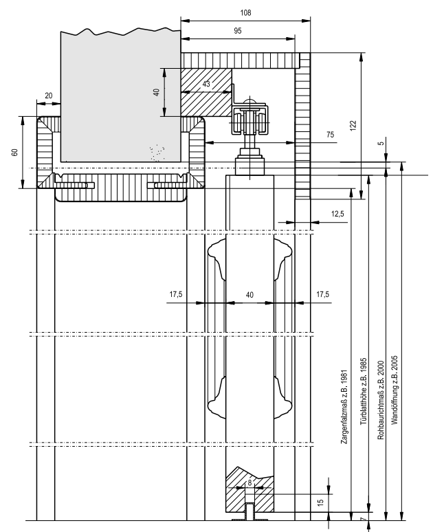
GARANT stilna drsna vrata tekoča pred steno
