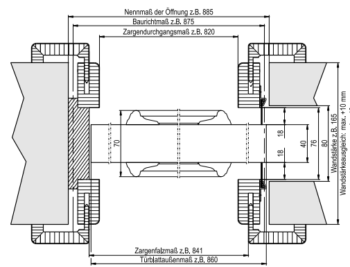
GARANT drsna vrata 2-krilna, varianta s kontraprofilom
