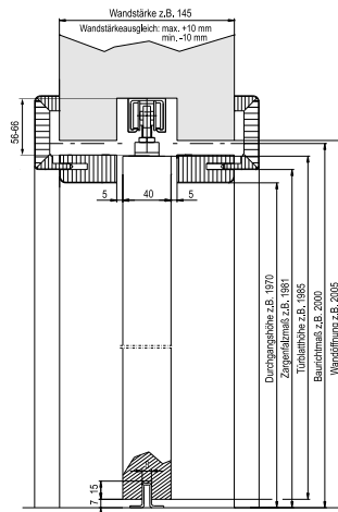
GARANT drsna vrata tekoča v steno
