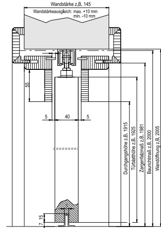
GARANT drsna vrata s svetl. izrezom v tekoča v steno
