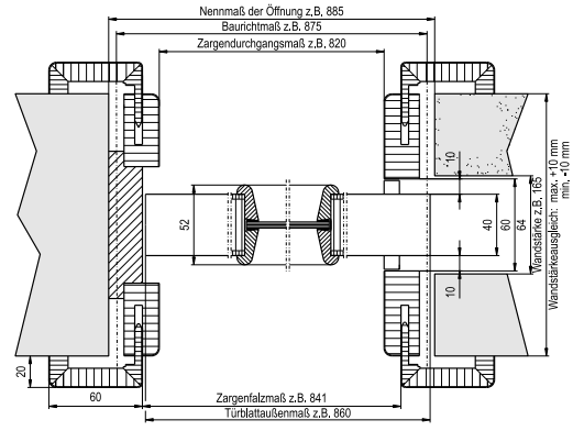
GARANT stilna drsna vrata v steno tekoča, varianta s ščetkastim tesnilom
