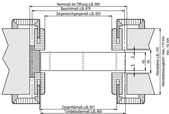
GARANT stilna drsna vrata v steno tekoča, standard
