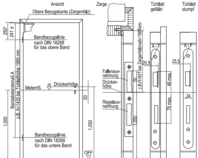
* Distanca od sredine nasadila do zgornjega roba krila A - F = Prislon do zadnjega roba jezika ključavnice
