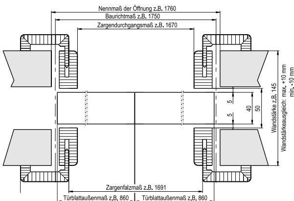
GARANT drsna vrata 2-krilna, standard
