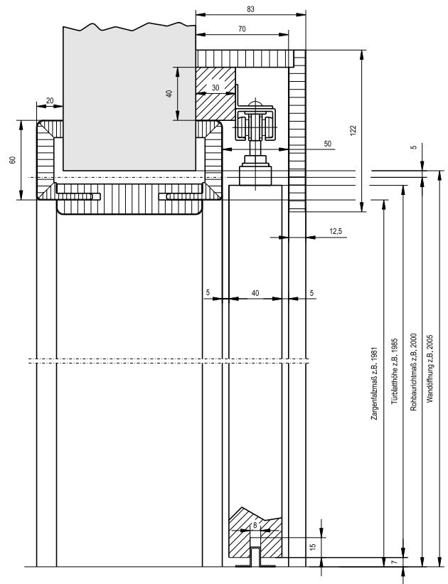
GARANT drsna vrata tekoča pred steno
