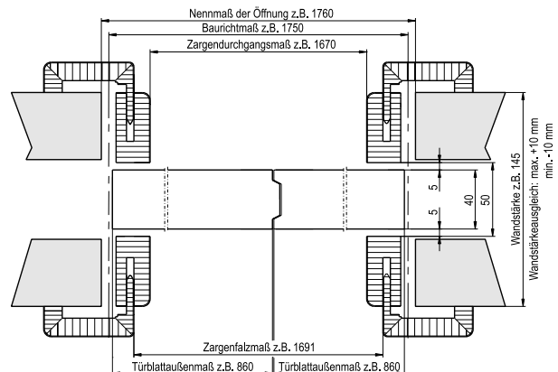
GARANT drsna vrata 2-krilna, varianta s kontraprofilom
